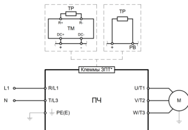
Рис. 3.2.3 — Подключение силовых клемм для моделей LCI-GY/PY-3
