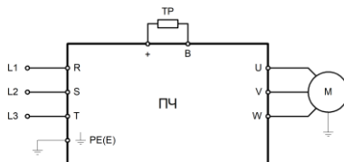
Рис. 3.2.4 — Подключение силовых клемм для моделей LCI-GY/PY-4B(S)
