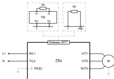
Рис. 3.2.2 — Подключение силовых клемм для моделей LCI-GY/PY-2(B)
