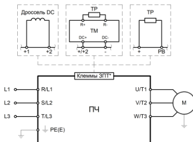
Рис. 3.2.5 — Подключение силовых клемм для моделей LCI-GY/PY-4(B)
