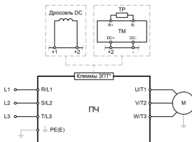
Рис. 3.2.6 — Подключение силовых клемм для моделей LCI-GY/PY-6
