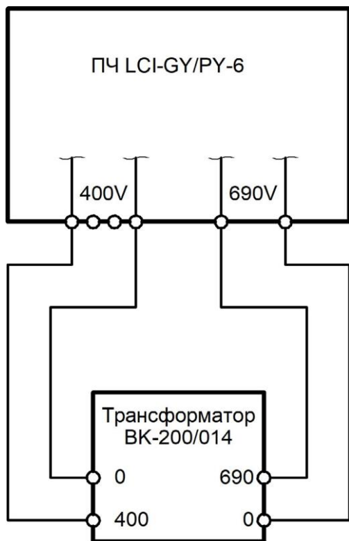
Рис. 3.2.7 – Схема подключения разделительного трансформатора для моделей LCI-GY/PY-6
