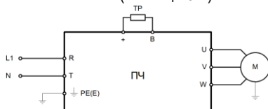
Рис. 3.2.1 — Подключение силовых клемм для моделей LCI-GY/PY-1 и LCI-GY/PY-2B(S)
